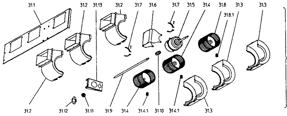
31 FAN ASSY
